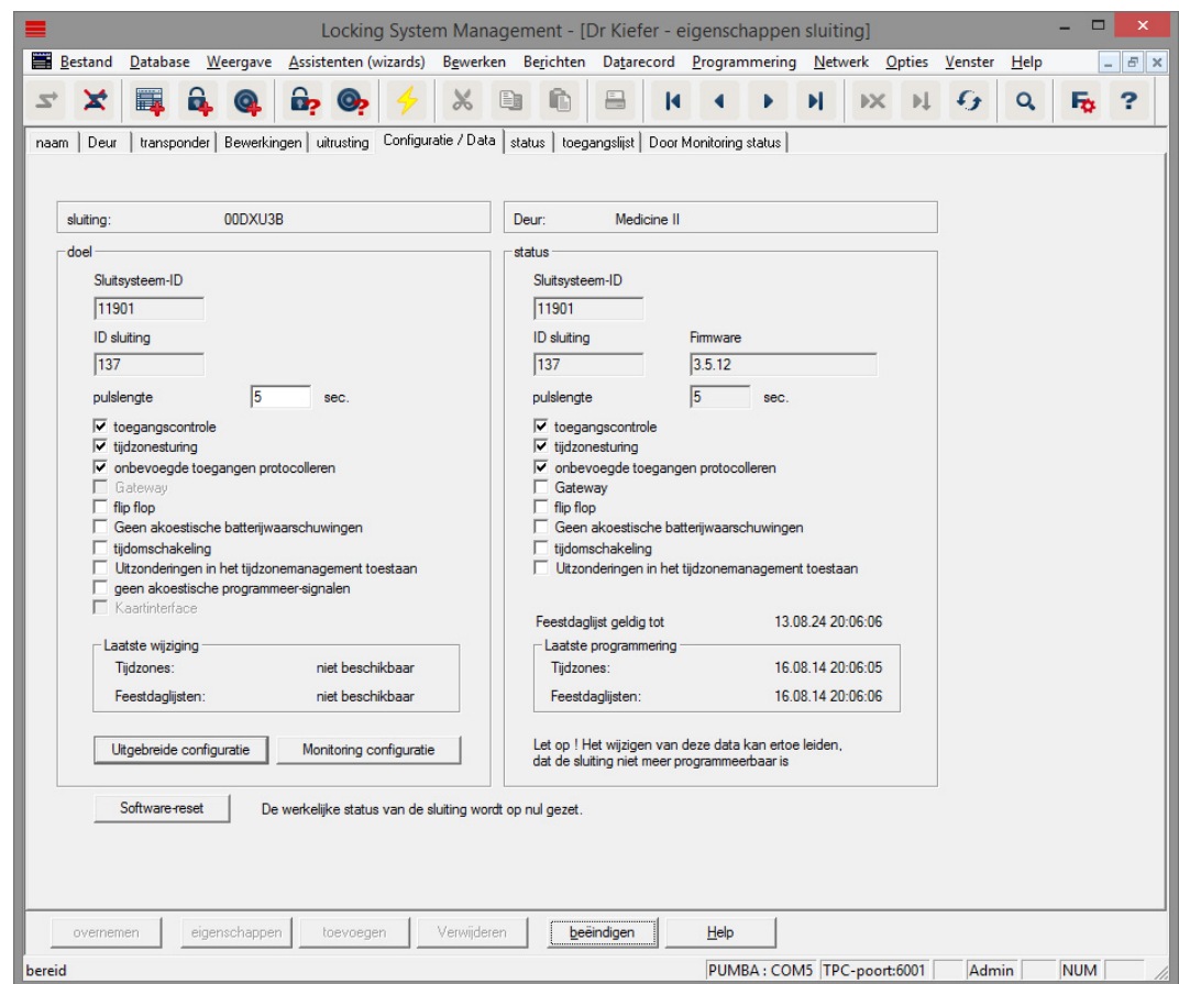
Afb. 8: Register 'Configuratie/gegevens'
