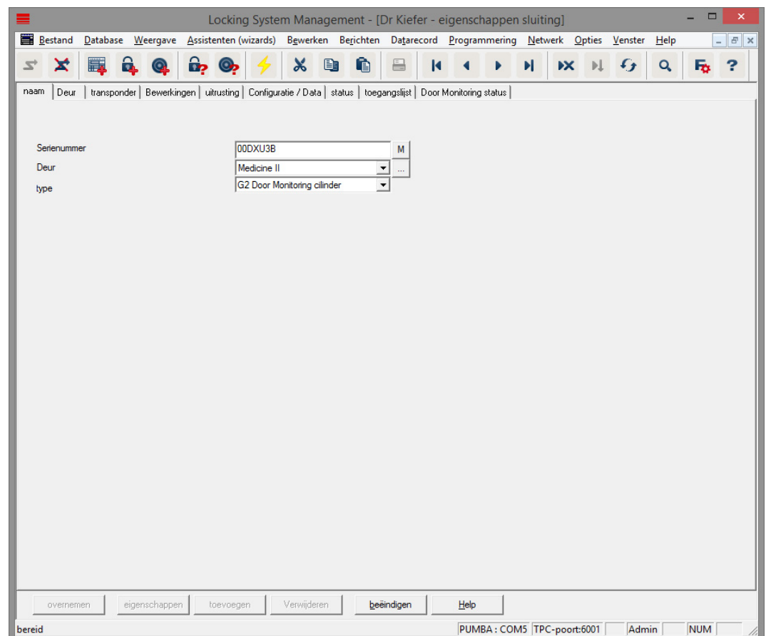
Afb. 3: Register 'Naam'
