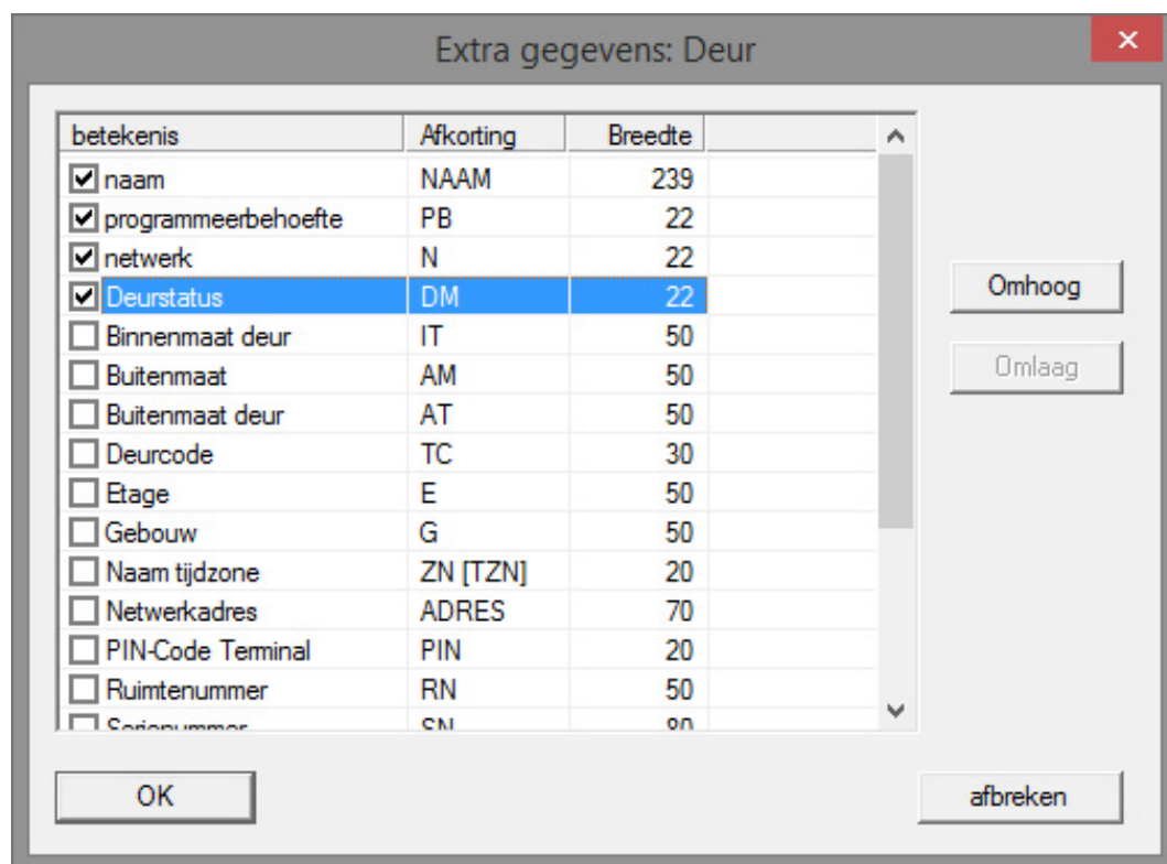
Afb. 15: Selectie kolommen
